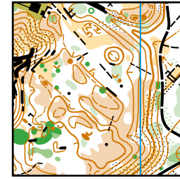
E4 1 : 10 000 e = 5 m
